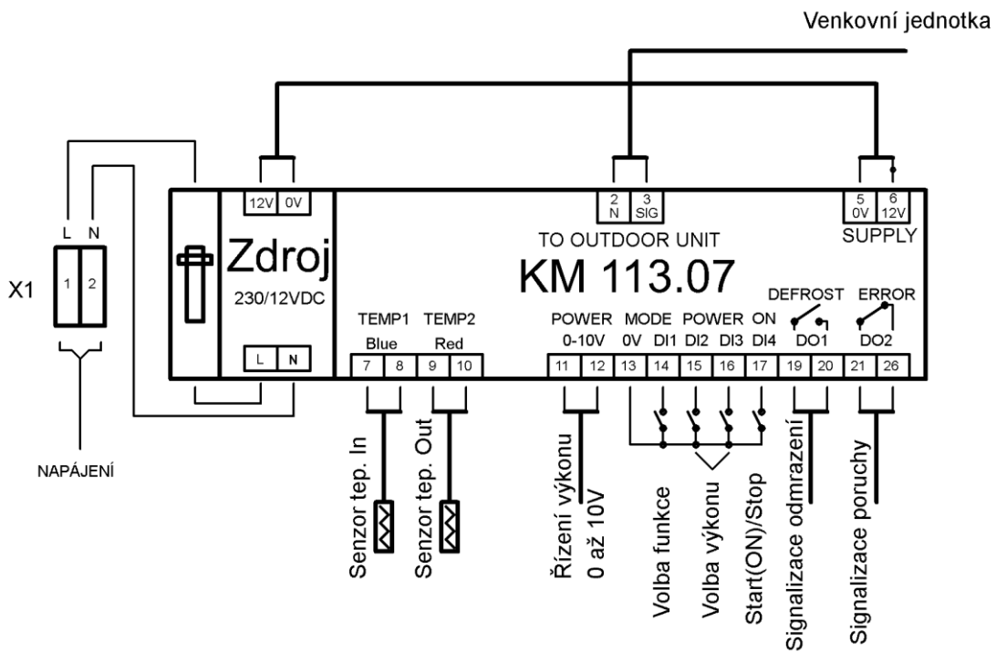
CELKOVÉ SCHÉMA SVOREK KM113.07UU (obr.4)
