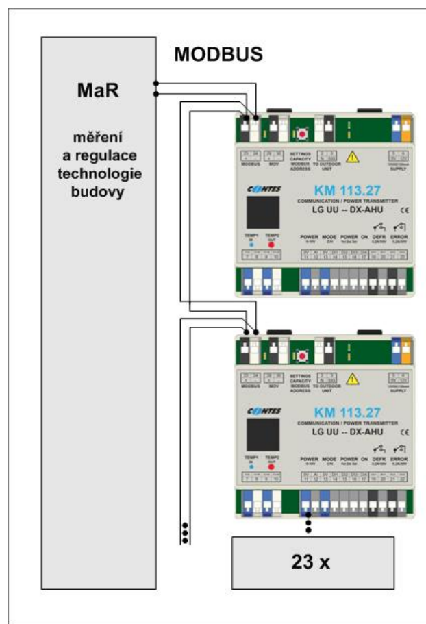
Obr.9 SCHÉMA ZAPOJENÍ KOMUNIKACE MODBUS PRO OVLÁDÁNÍ VÍCE MODULŮ
