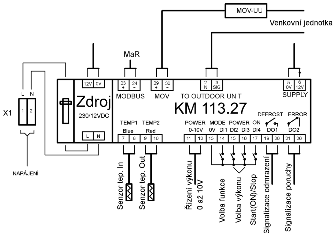
CELKOVÉ SCHÉMA SVOREK KM113.27UU (obr.2 )
