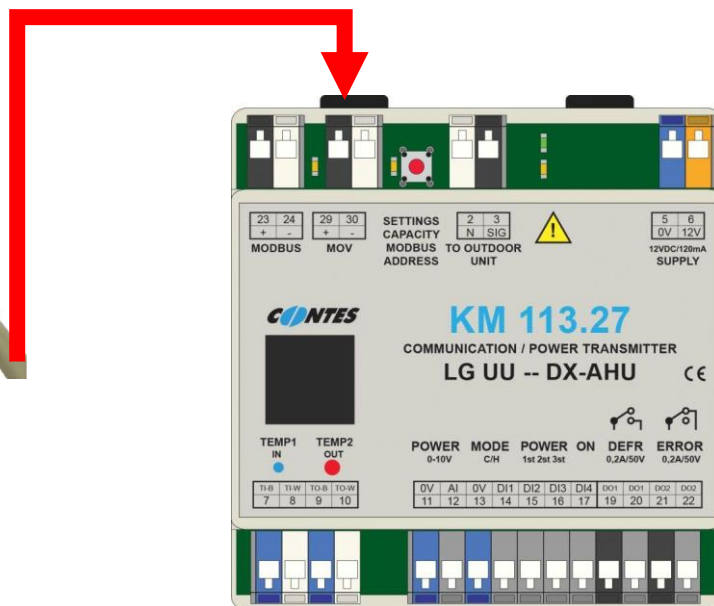
SCHÉMA PŘIHOJENÍ MOV-UU ke kompresorové jednotce UU-- + modulu KM113.27UU (obr.6) (příklad pro jednotku UU18W.UE4)
