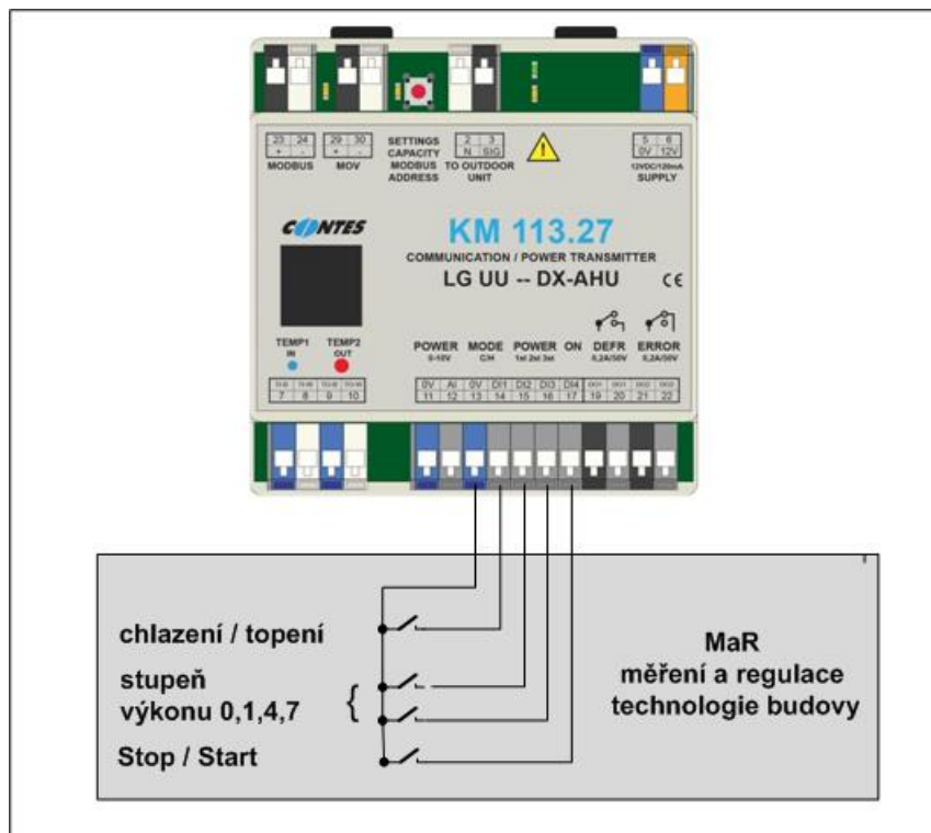
SCHÉMA OVLÁDÁNÍ LOGICKÝMI VSTUPY (obr.8)
